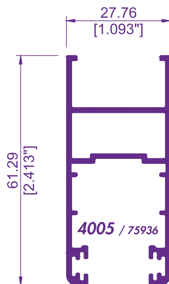
HOJA PERIMETRAL DOBLE VIDRIO
