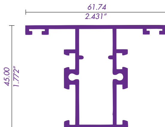
4521 / 62041 INTERMEDIO CUADRÍCULA
