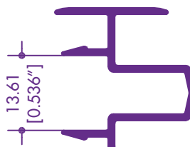
8043 / 62103 ADAPTADOR OXXO
