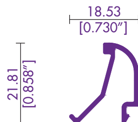
8023 / 82030 JUNQUILLO 24mm.
