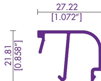
8022 / 82029 JUNQUILLO 6mm.
