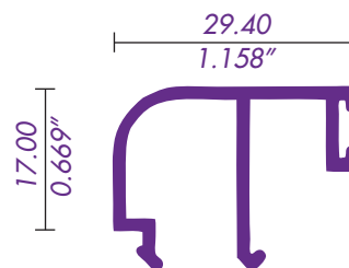
4594 / 62029 JUNQUILLO 6mm.
