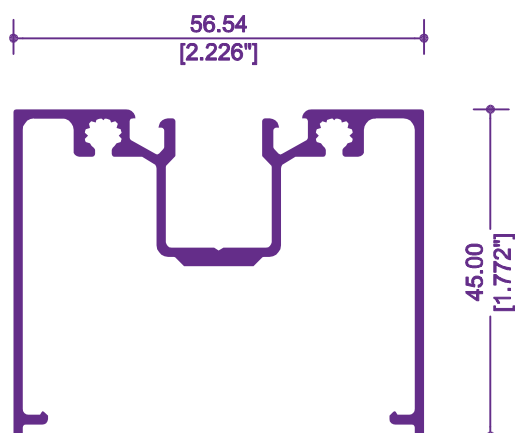
5025 / 12504 BOLSA
