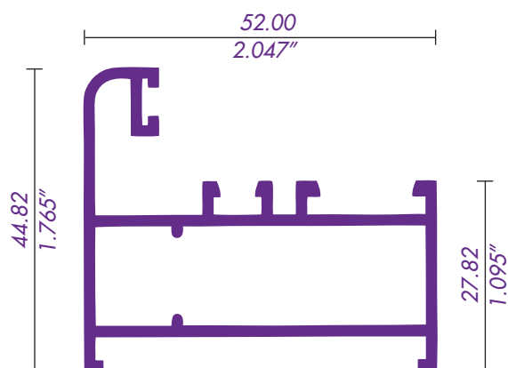
4525 / 62033 "L" CONTRAMARCO
