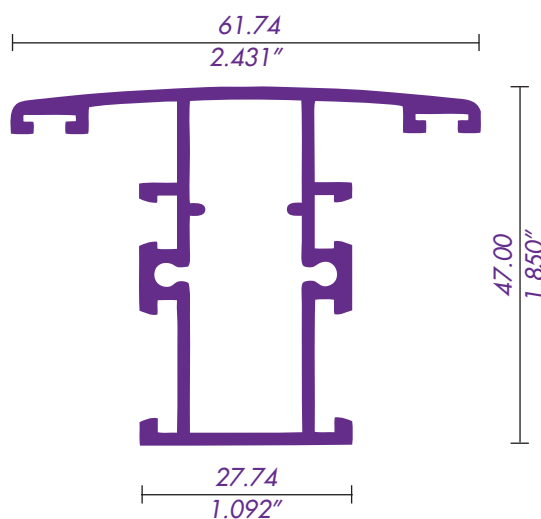
4524 / 62028 "T" INTERMEDIO
