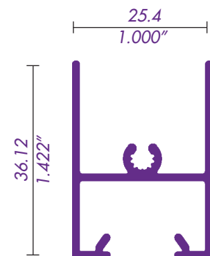
315 / 67836 CABEZAL VENTANA
