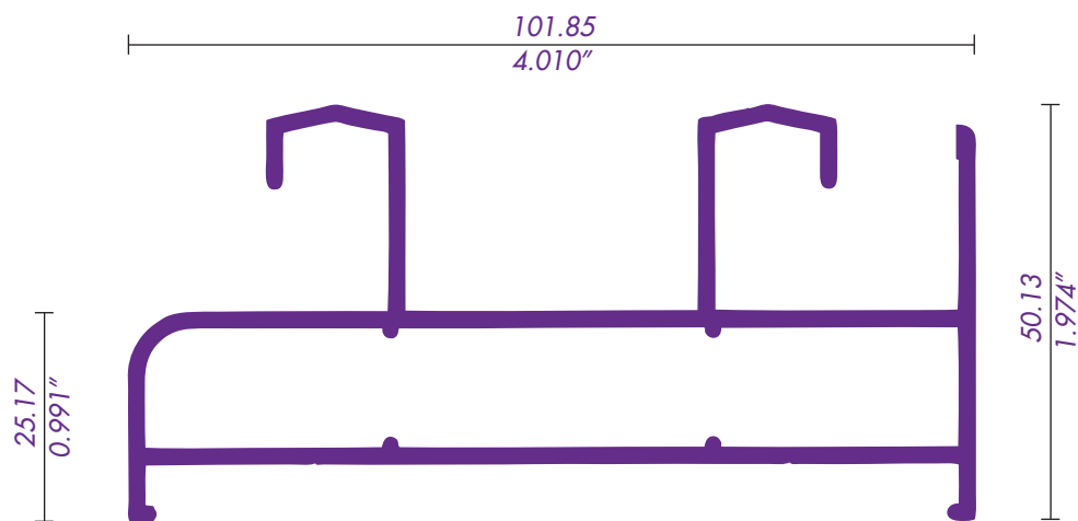
1519 / 62052 RIEL DOBLE
