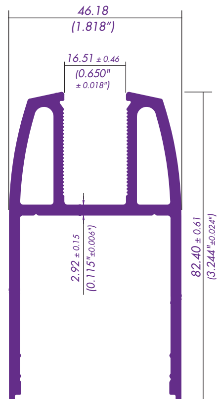
688 / 75673 ZOCLO HERCULITE LIGERO TAPA ZOCLO 829/PN-0929
