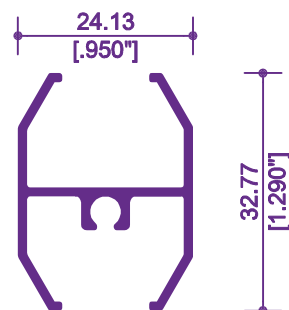
7086 / 14918 PERFIL P/CUADRÍCULA
