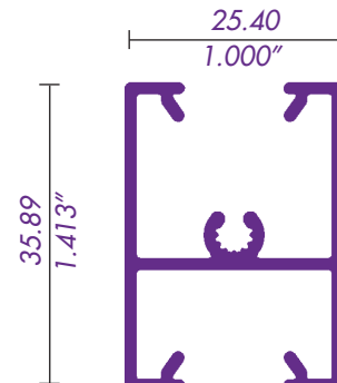
305 / 69082 INTERMEDIO
