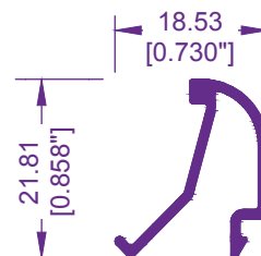
8023 / 82030 JUNQUILLO
