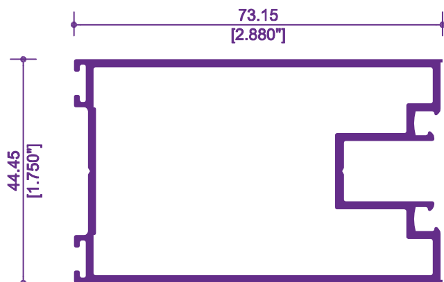
5096 / 14386 CERCO CON JUNQUILLO INTEGRADO
