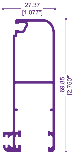
6012 / 68299 MOSQUITERO EXT.
