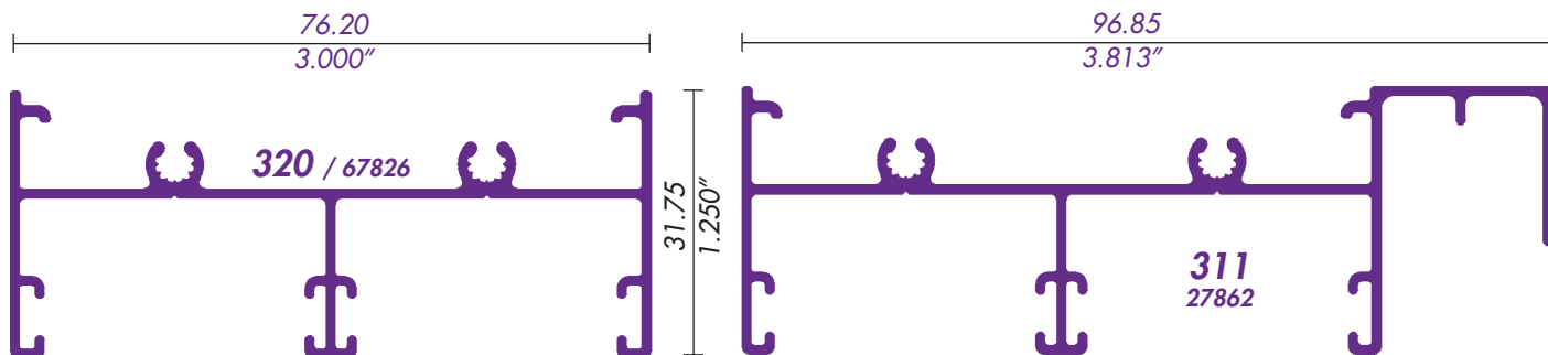
CABEZAL Y JAMBA
