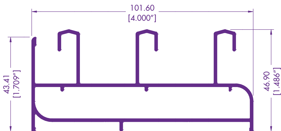
8029 / 82017 RIEL TRIPLE
