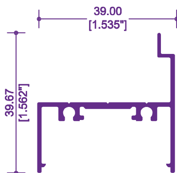
3505 / 13363 CONTRAMARCO
