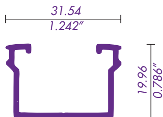
1516 / 62060 ADAPTADOR CRIS- TAL 9mm
