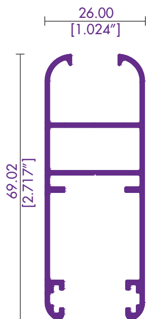
8017 / 82001 CERCOS 6mm
