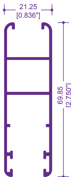
6014 / 67894 CERCO 2.75\"/>
