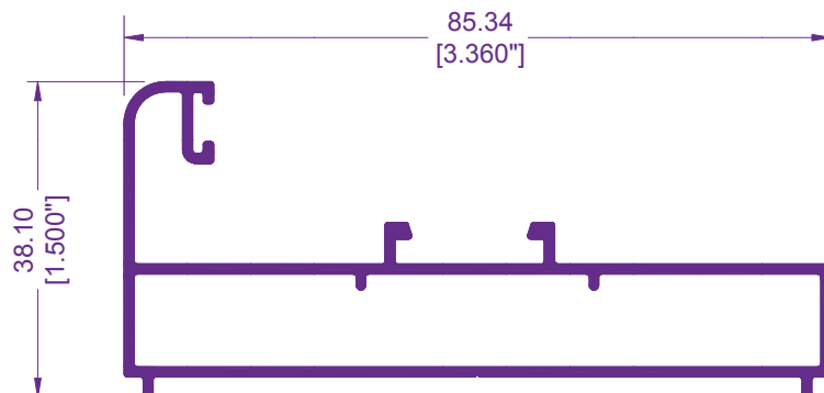
6021 / 82093 ESCALONADO DOS VIAS CON MOSQ.
