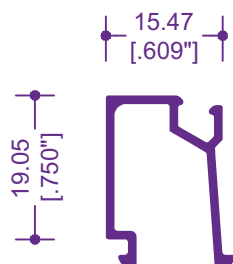
5093 / 12543 JUNQUILLO
