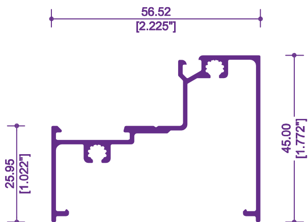
5022 / 12506 ESCALONADO EXTERIOR
