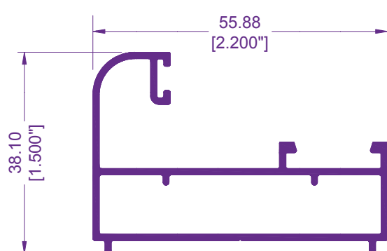
6024 / 82079 ESCALONADO
