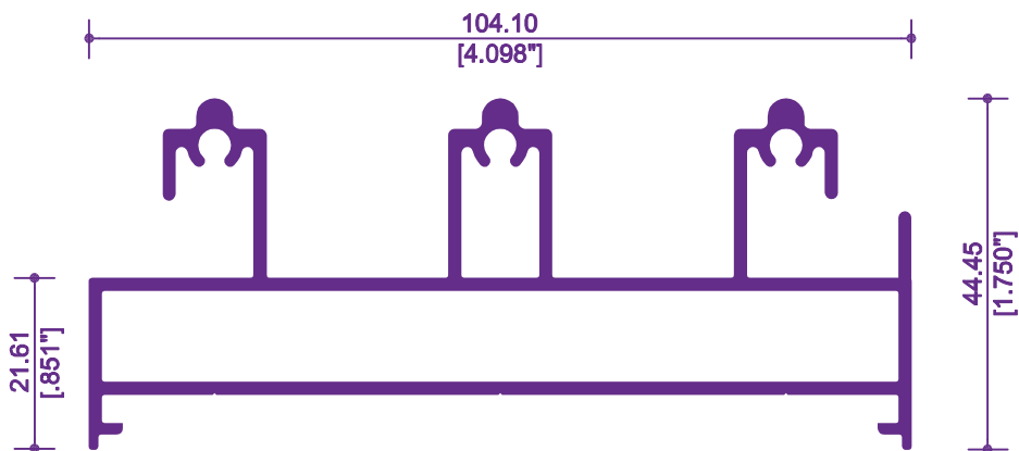
7059 / 72373 RIEL TRIPLE
