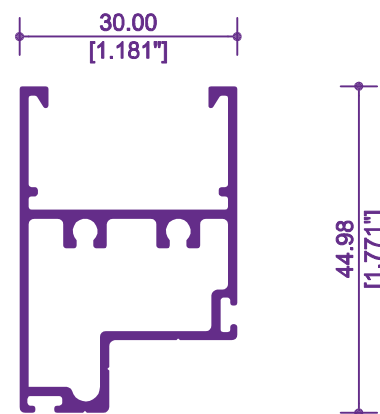
3506 / 12277 MARCO DOBLE VIDRIO
