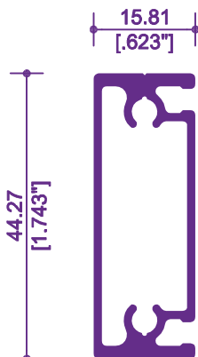
7084 / 11411 MOSQUITERO
