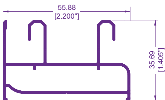
6019 / 87896 RIEL DE DOS PISTAS
