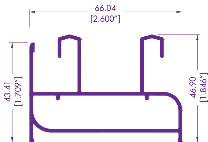
8019 / 82000 RIEL BASICO
