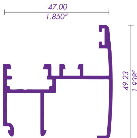
4528 / 62031 INTERMEDIO MOVIL
