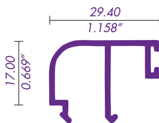
4594 / 62029 JUNQUILLO 6mm.
