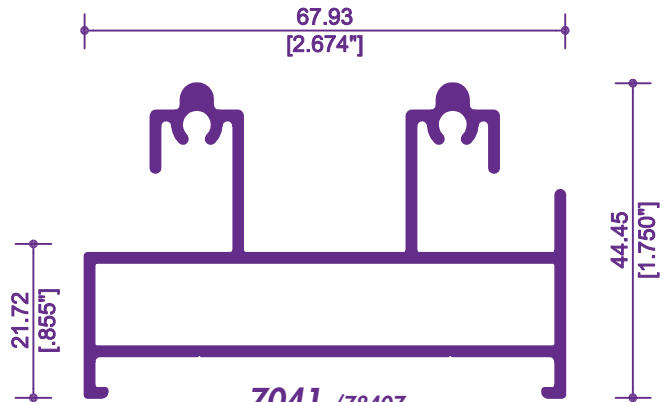
7041 / 78407 RIEL-CABEZAL
