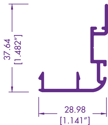
8018 / 82002 TRASLAPE
