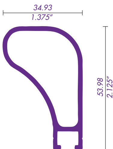
8034 / 62014 REFUERZO
