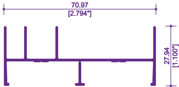
7040 / 78408 JAMBA
