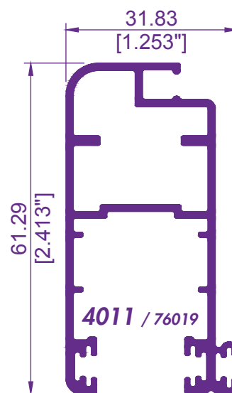
HOJA PERIMETRAL MOSQUITERO
