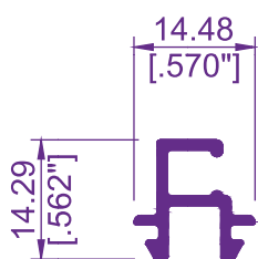
4006 / 76014 ADAPTADOR MOSQUITERO
