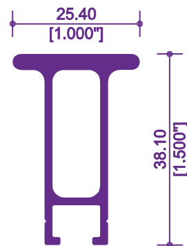
7038 / 14411 REFUERZO 1 1/2"
