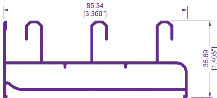
6020 / 88300 RIEL TRIPLE MOSQUITERO
