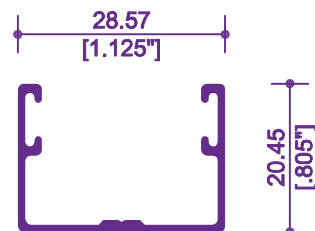
7082 / 18413 GUÍA INFERIOR
