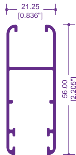
6017 / 62066 CERCO VENTANA
