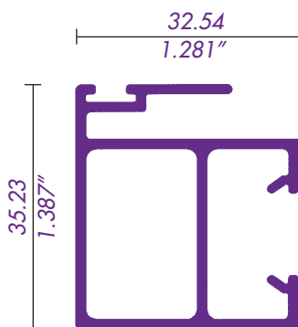
308 / 67844 CERCO TRASLAPE VENTANA
