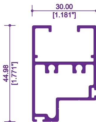
3504 / 12276 MARCO
