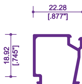
5023 / 12507 JUNQUILLO
