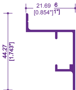
7080 / 11409 CABEZAL MOSQUITERO
