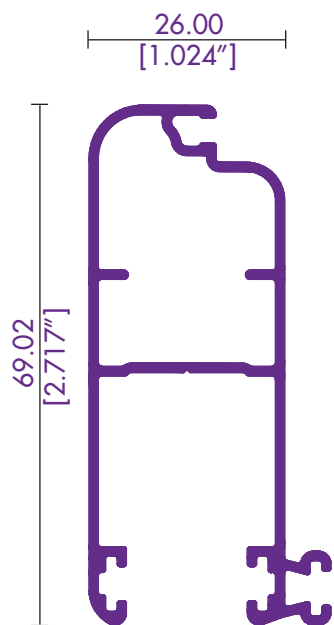
8012 / 82019 MOSQUITERO DE LUJO
