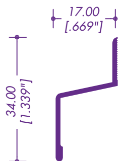
7081 / 12428 BOTAGUAS EUROVENT
