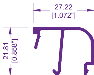
8022 / 82029 JUNQUILLO
