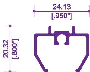
7085 / 14702 PERFIL P/CUADRÍCULA
