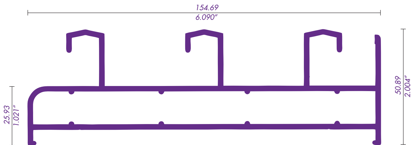
1529 / 62054 RIEL TRIPLE
