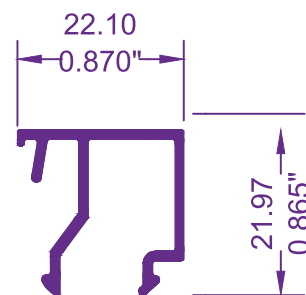
4012 / 76095 JUNQUILLO P/FIJO TUBULAR
