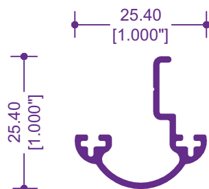
5084 / 12653 ADAPTADOR INTERMEDIO
