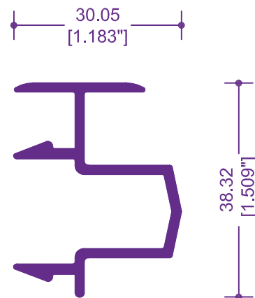
1543 / 64206 ADAPTADOR OXXO
