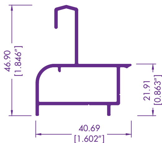
8021 / 84207 ADAPTADOR RIEL
