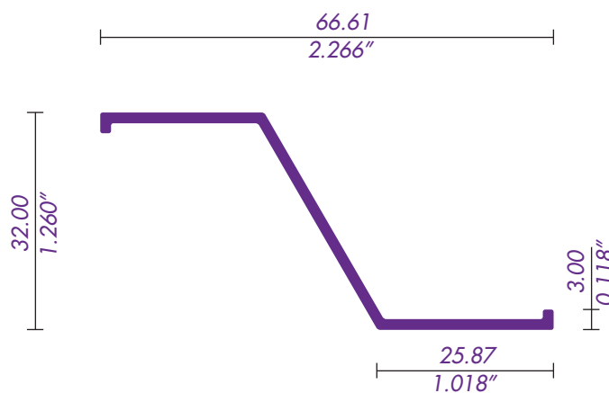
259 / 63299 CELOSIA Z 2.6"
