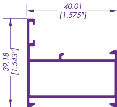
1602 / 73971 CERCO LISO VENTANA
