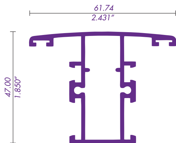
4525 / 62033 "L" CONTRAMARCO
