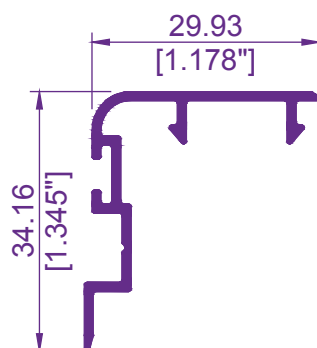
4003 / 75826 TAPA HOJA CENTRAL
