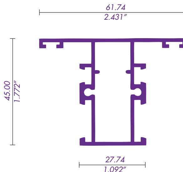
4521 / 62041 INTERMEDIO CUADRICULA
