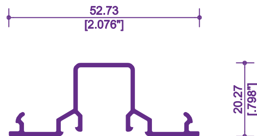
5027 / 12505 TAPA BOLSA
