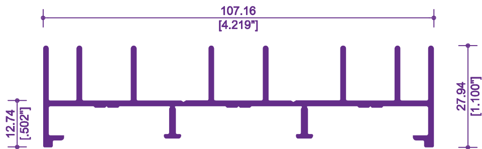
7050 / 62374 JAMBA
