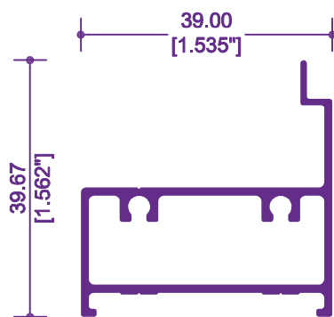
3501 / 12273 CONTRAMARCO
