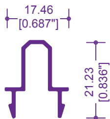
6006 / 62078 ADAPTADOR XX
