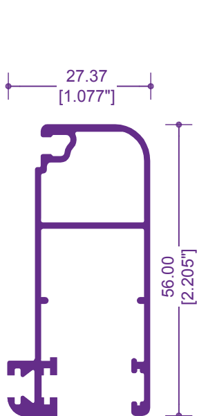
6011 / 68337 MOSQUITERO BAJO
