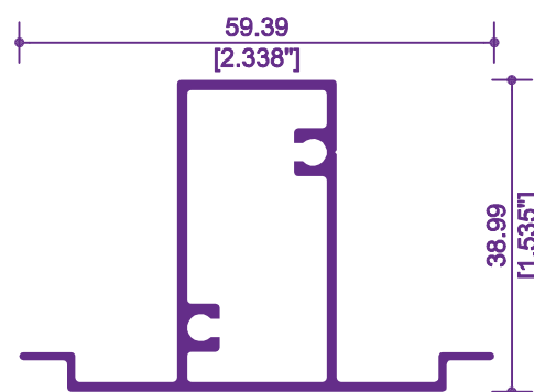
3502 / 12275 INTERMEDIO
