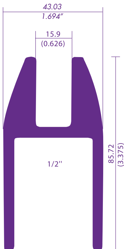
689 / 68327 ZOCLO HERCULITE
