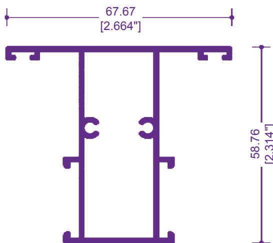
8015 / 62047 INTERMEDIO FIJO PLANO
