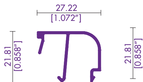
8022 / 82029 JUNQUILLO 6mm.
