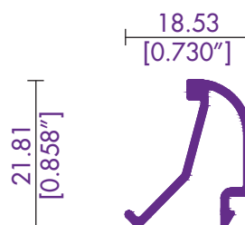
8023 / 82030 JUNQUILLO 24mm.
