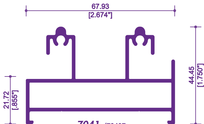
7041 / 78407 RIEL-CABEZAL
