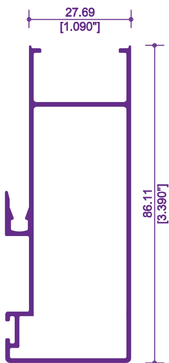
7078 / 78420 TRASLAPE DOBLE VIDRIO
