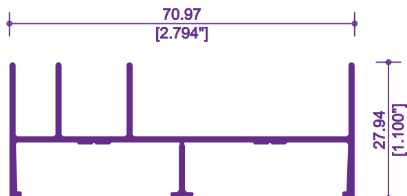
7040 / 78408 JAMBA
