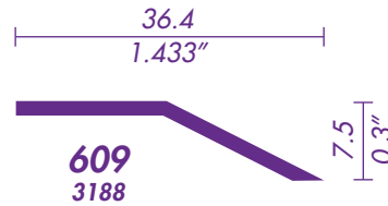
MOLDURA DE ALFOMBRA
