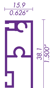
212 / 10358 MOSQUITERO CORREDIZO
