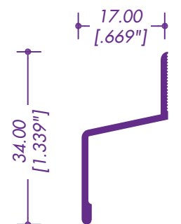
7081 / 12428 BOTAGUAS EUROVENT
