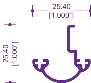
5084 / 12653 ADAPTADOR INTERMEDIO
