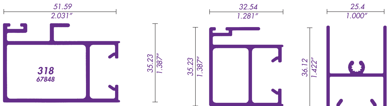
TRASLAPE PUERTA 352 en 610
