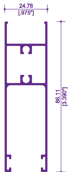
7076 / 12437 ZOCLO-CABEZAL DOBLE VIDRIO
