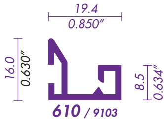
MOLDURA PARA MARCOS
