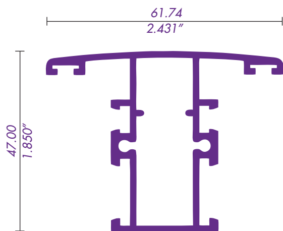
4525 / 62033 "L" CONTRAMARCO
