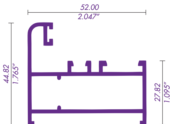
4525 / 62033 "L" CONTRAMARCO
