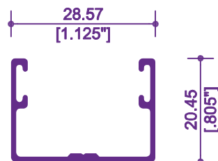
7082 / 18413 GUÍA INFERIOR
