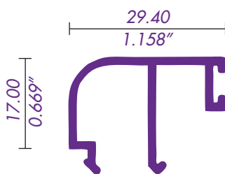
4594 / 62029 JUNQUILLO 6mm.
